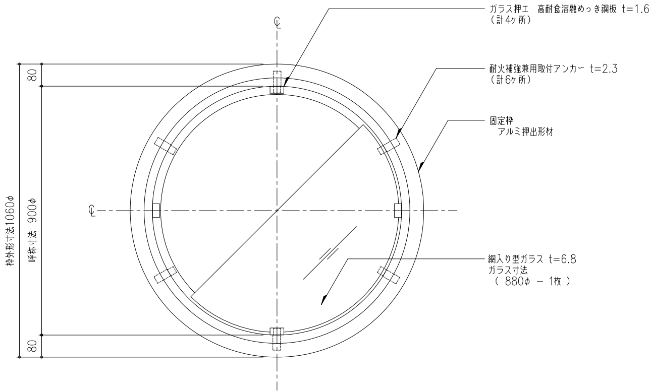
枠伏図 S=1:10
